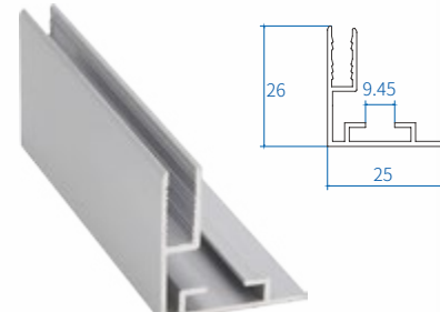
Size(H*W*wt) : 25.6 × 25 × 1.2
