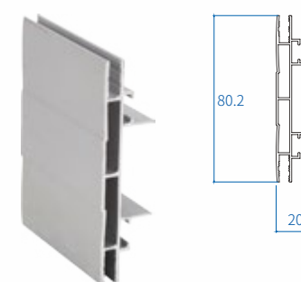
Size(H*W*wt) : 80.2 × 20 × 1.4
