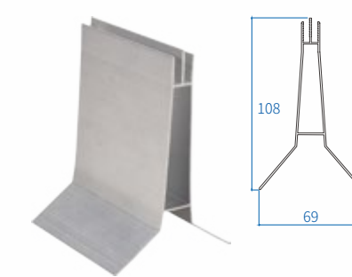
Size(H*W*wt) : 108 × 69 × 1.2
