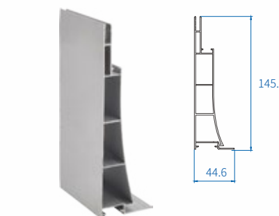
Size(H*W*wt) : 145.6 × 44.6 × 1.4
