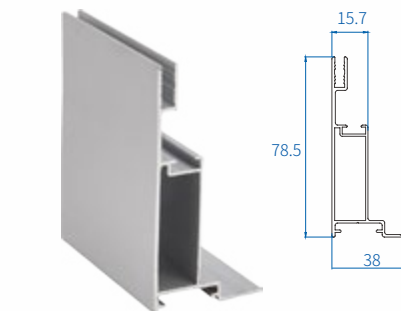
Size(H*W*wt) : 79 × 38.6 × 1.8
