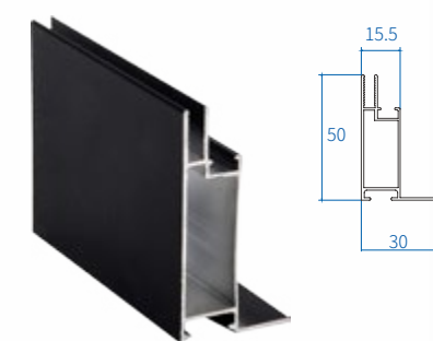
Size(H*W*wt) : 59.2 × 30 × 1.2
