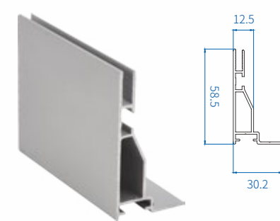
Size(H*W*wt) : 60.2 × 30.8 × 1.5
