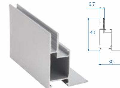
Size(H*W*wt) : 40 × 30 × 1.2
