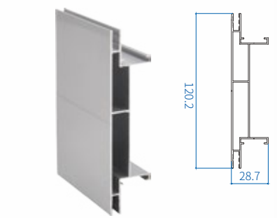
Size(H*W*wt) : 119.9 × 28.3 × 1.4
